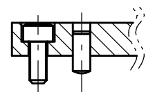
A-A矢視 A-A VIEW
