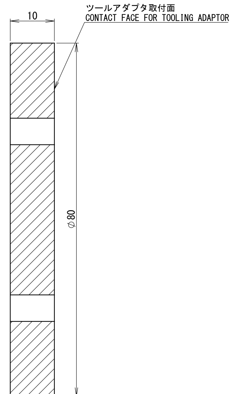
断面図 A-A SECTION A-A
