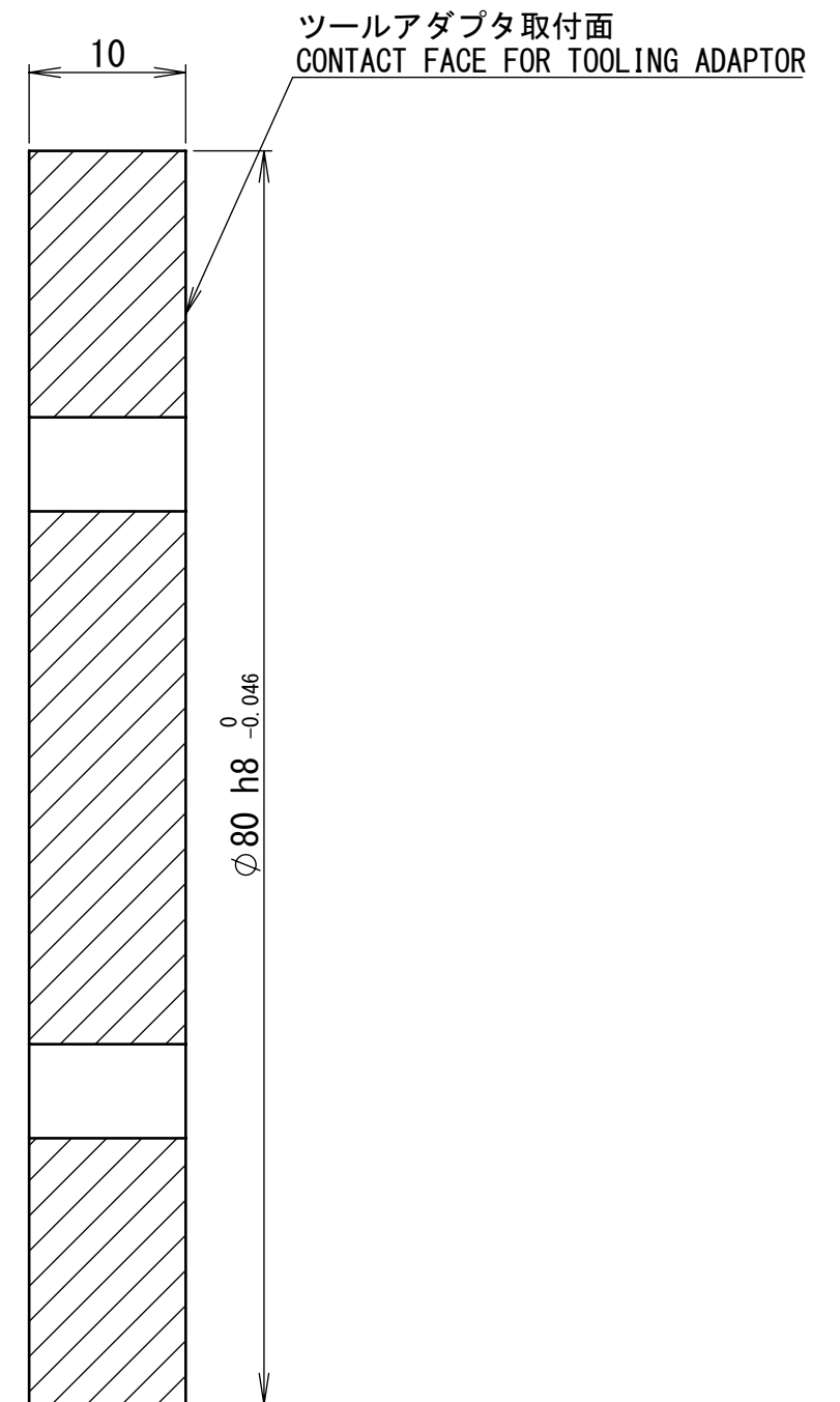
断面図 A-A SECTION A-A
