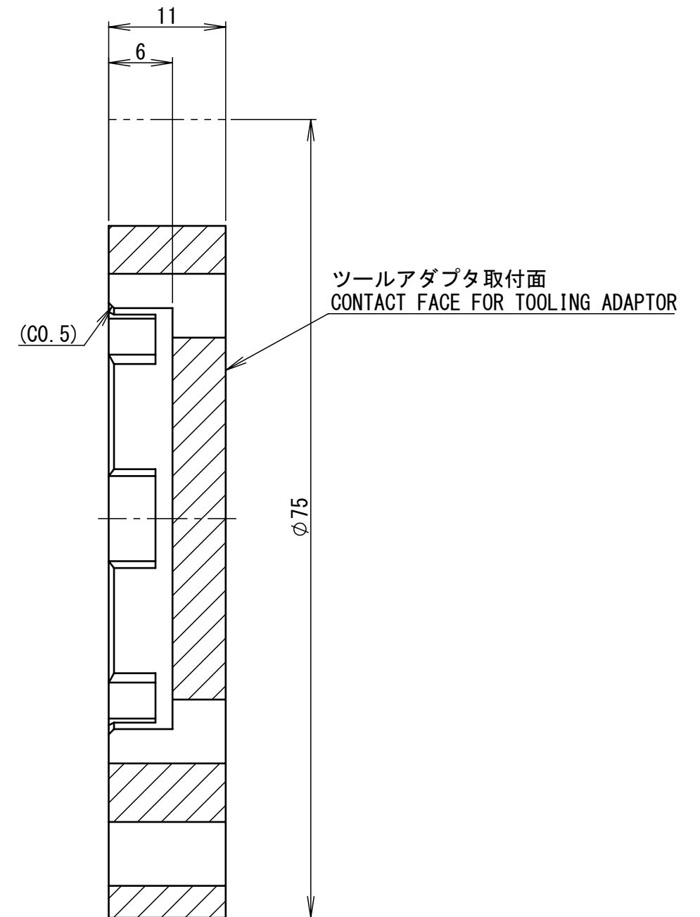
断面図 A-A SECTION A-A
