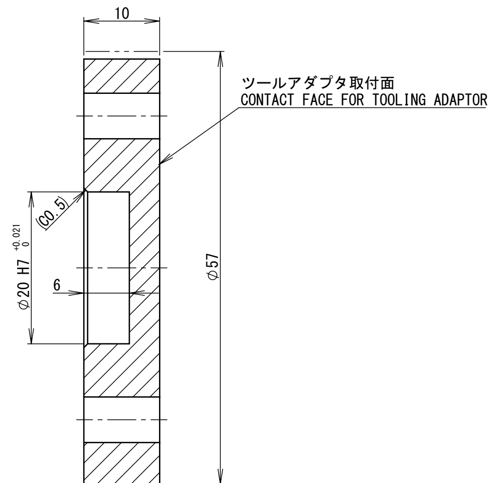
断面図 A-A SECTION A-A
