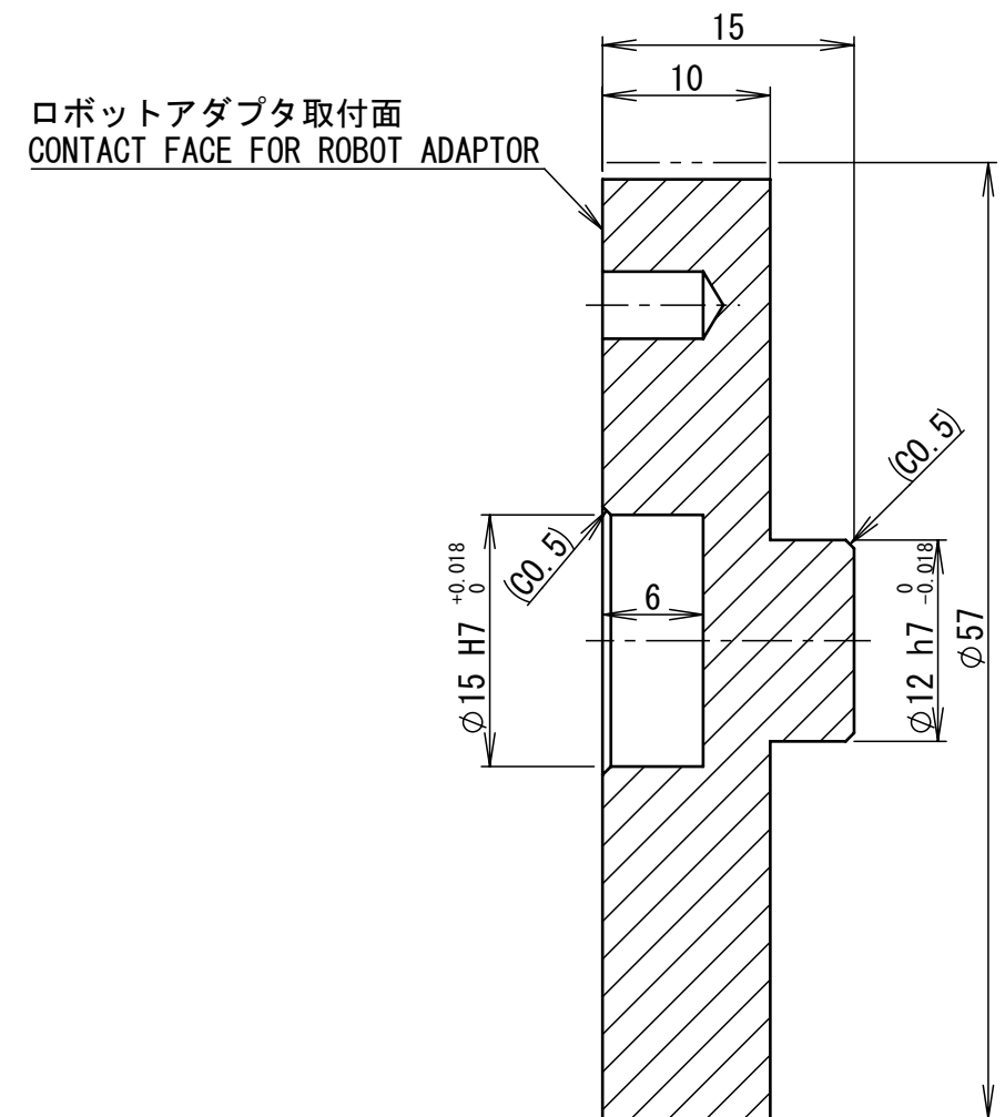
断面図 A-A SECTION A-A
