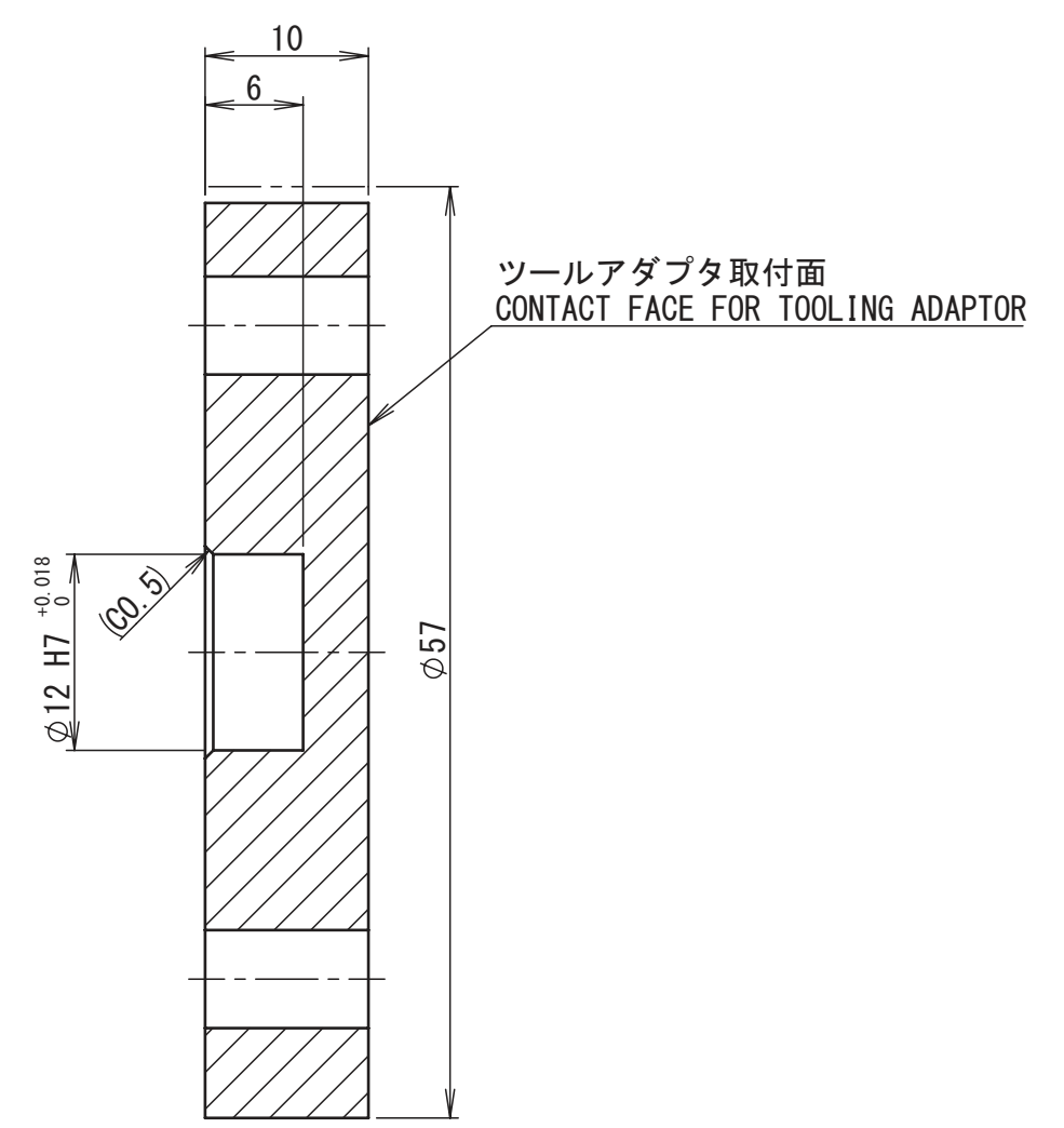
断面図 A-A SECTION A-A
