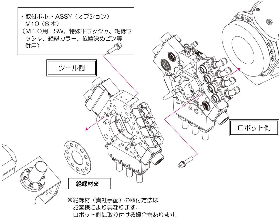
図 5. ロボットおよびツールの組立図
