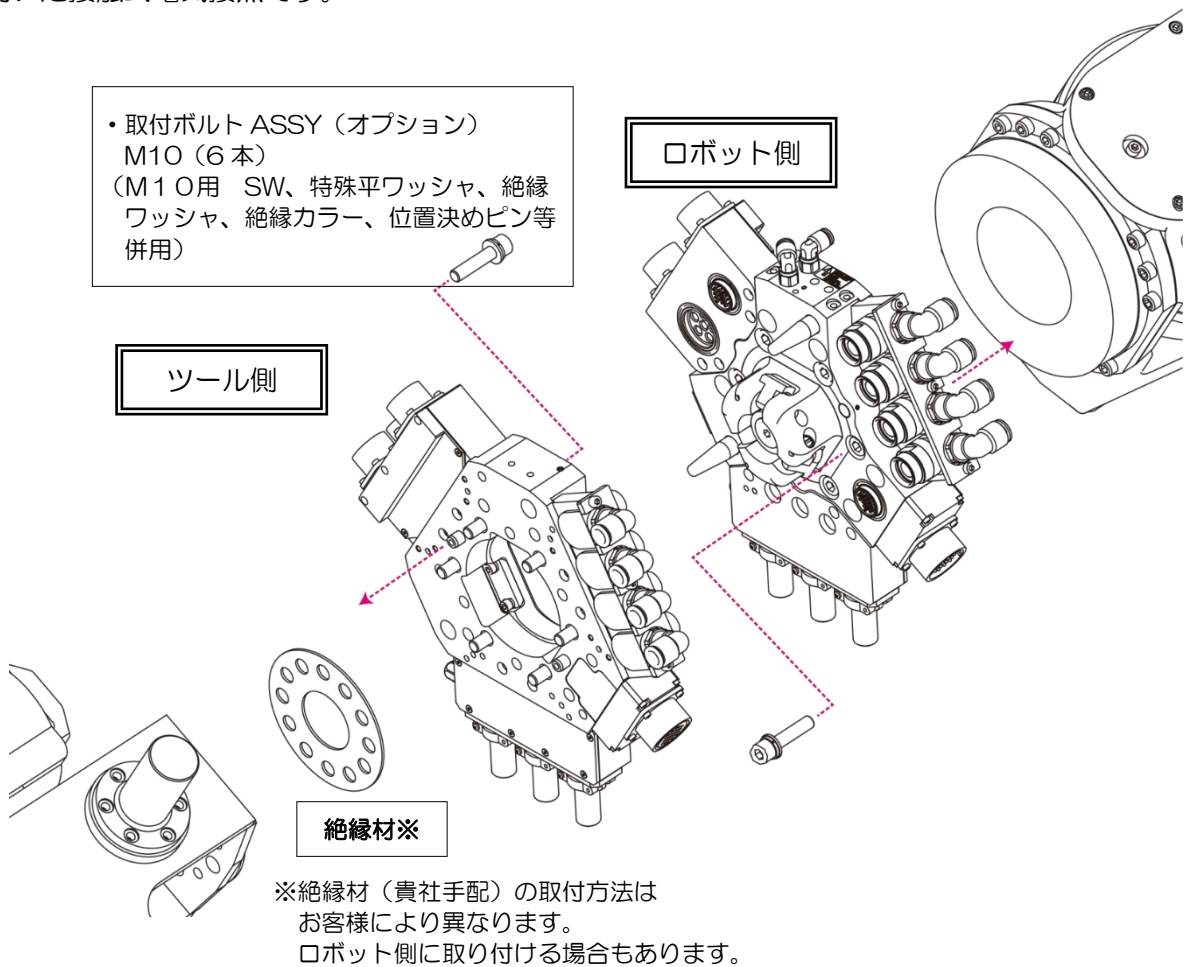
図 1.システム図
