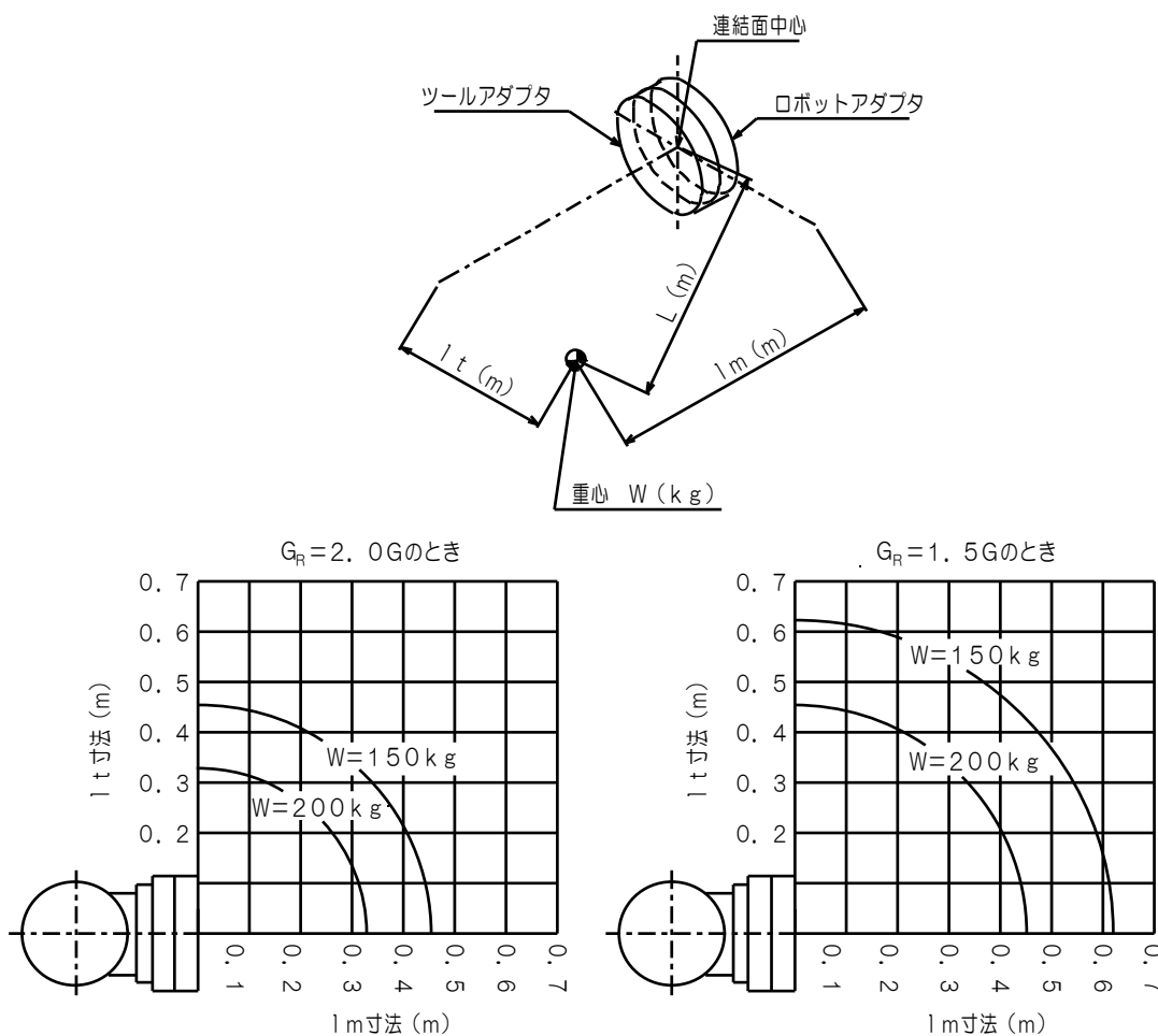
図 3. 定格負荷の定義一例 G_R=1.5, 2.0 の場合
