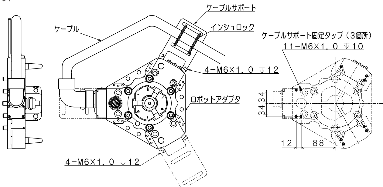
図 9. ケーブル固定方法の一例
