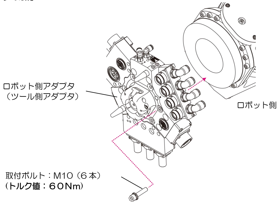
図 7. ロボットアダプタの取付
