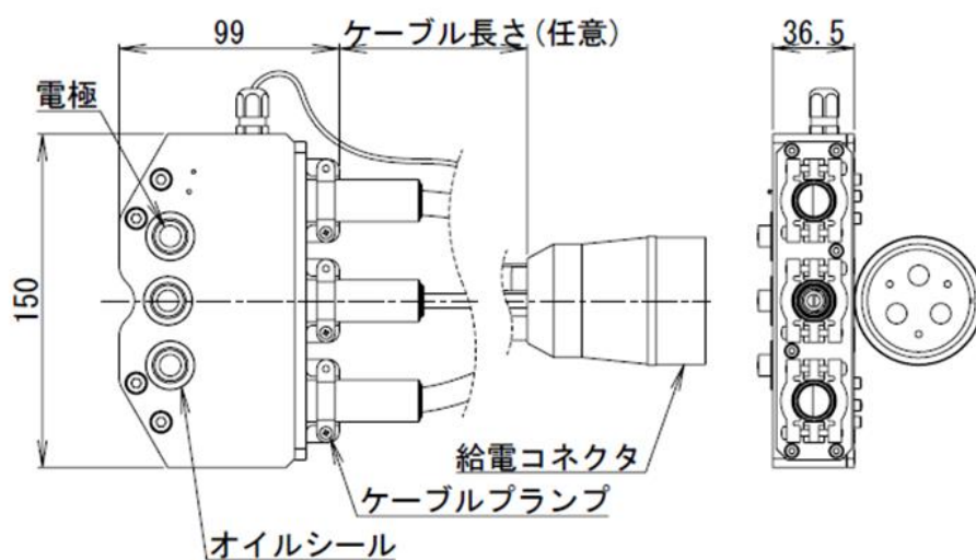
T側給電モジュール （詳細は納入仕様図 面参照のこと）
