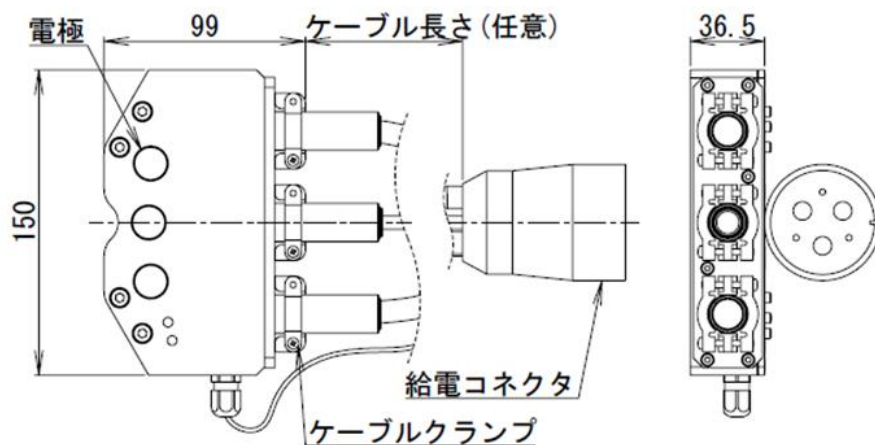
R側給電モジュール （詳細は納入仕様図 面参照のこと）
