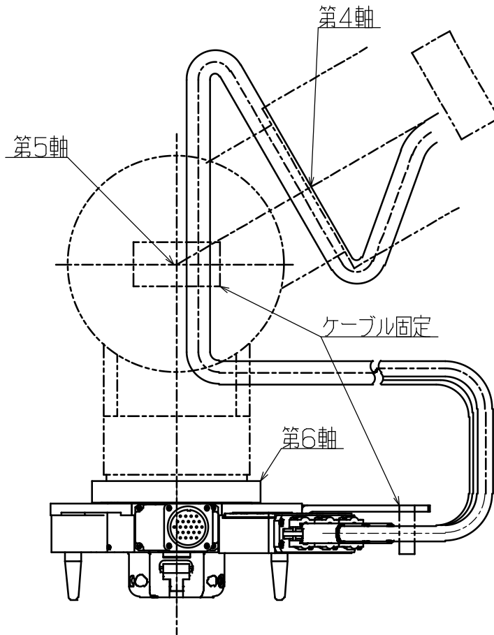
図 20. ケーブル固定方法の一例
