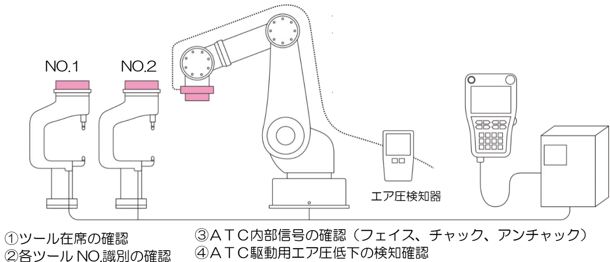
図 12. インターロックの例
