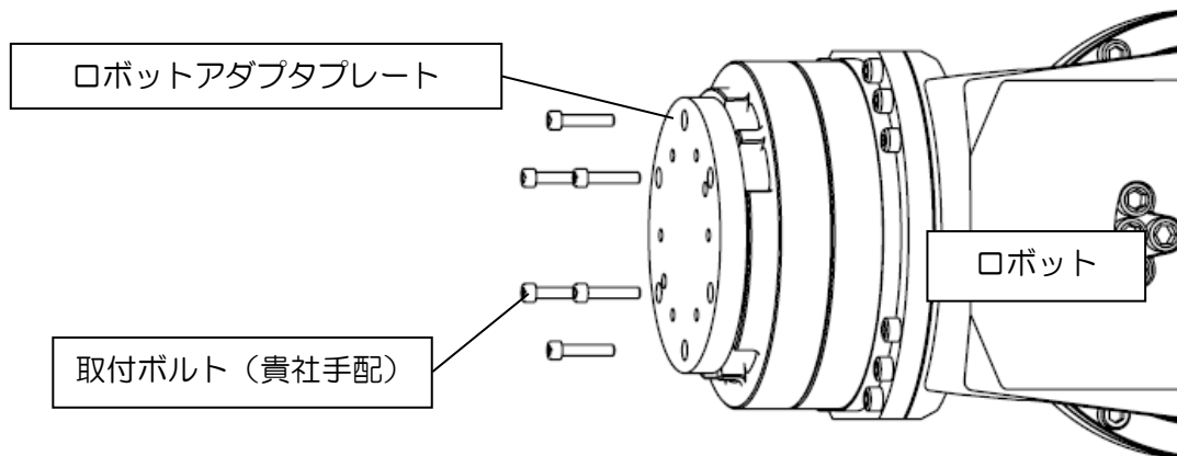
図 7.ロボットアダプタプレートの取付
