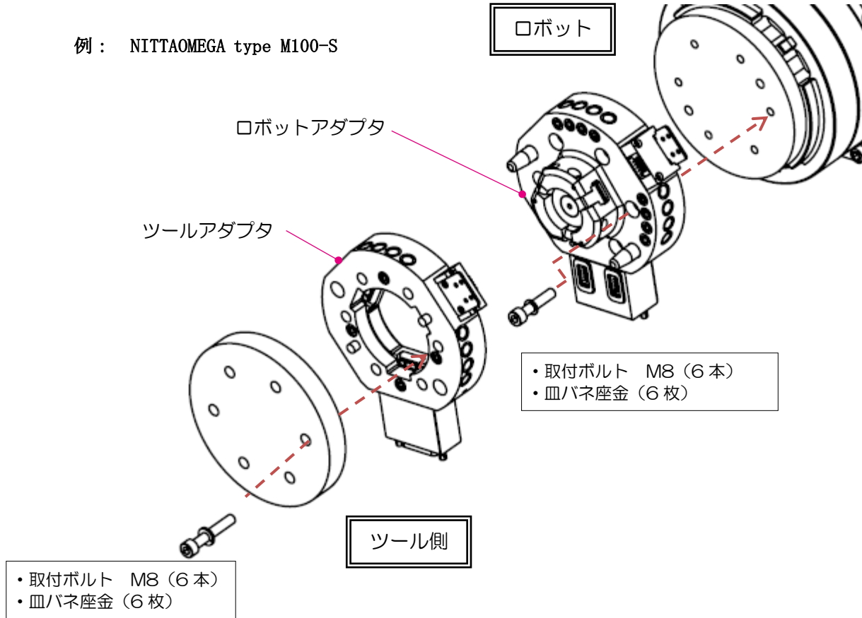
図 6. ロボットおよびツールの組立図
