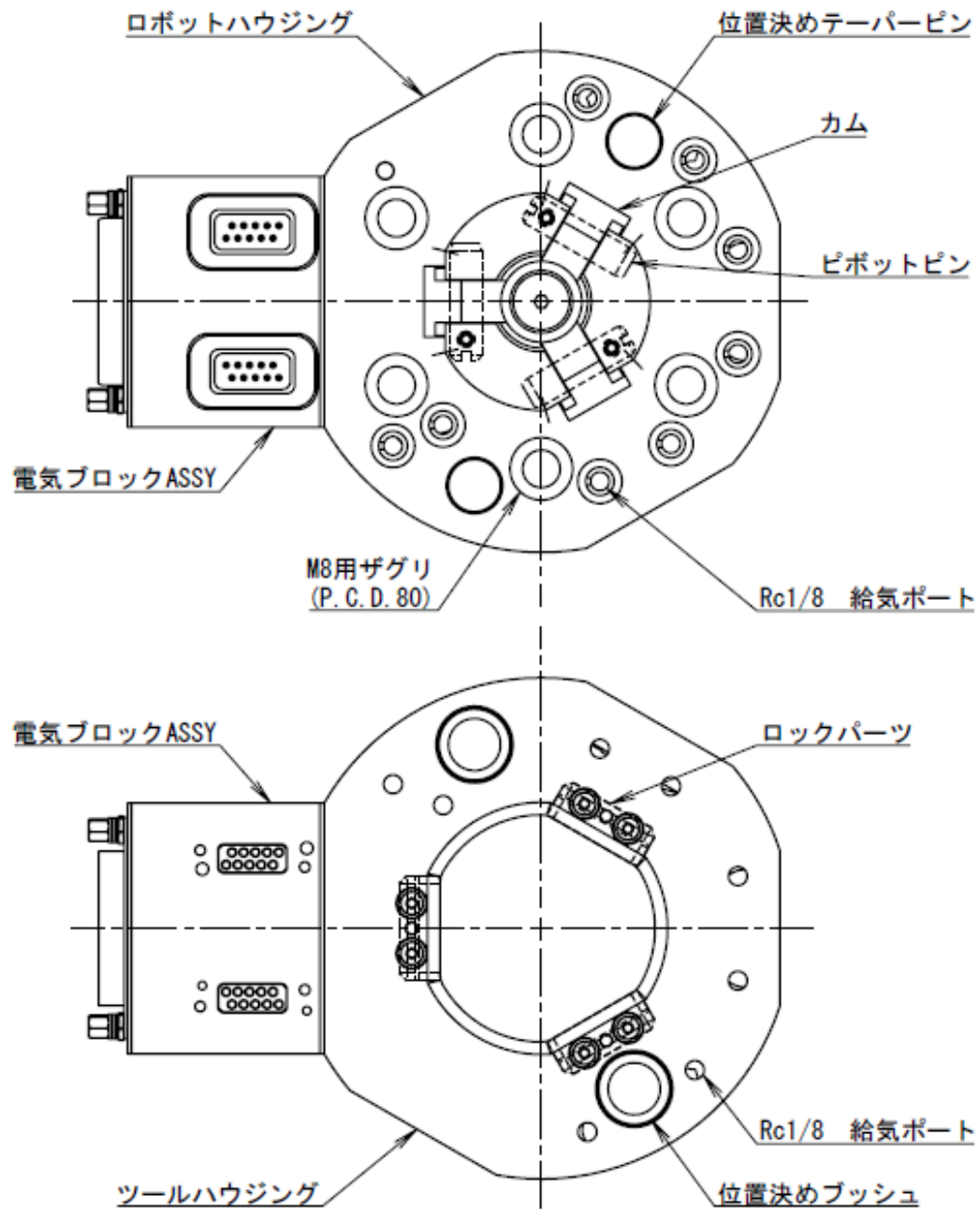
図3. typeS50-S 各部の名称
