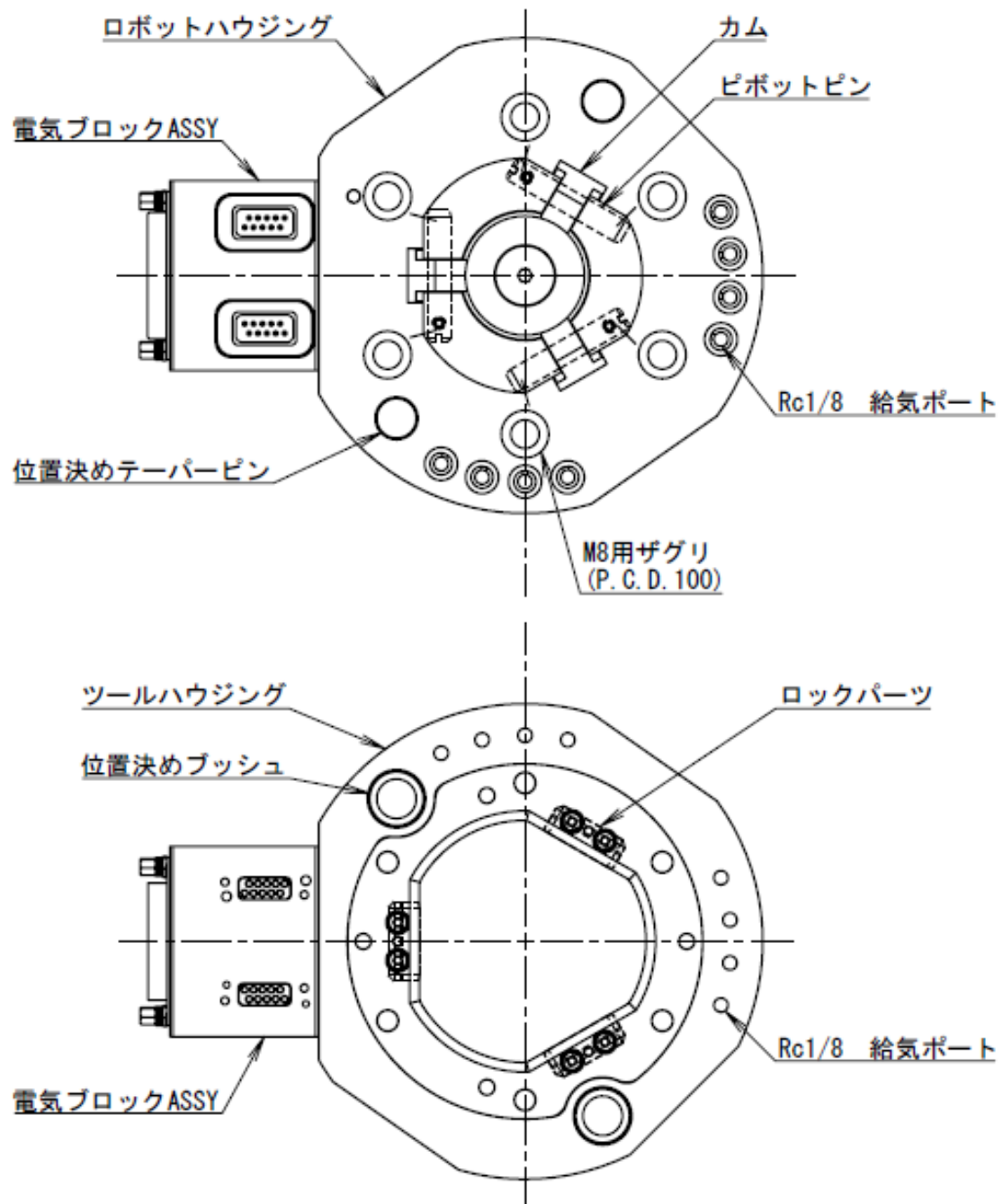
図2. type M100-S 各部の名称
