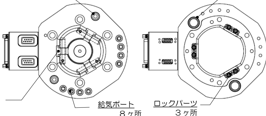
図 10. ATC給脂箇所
