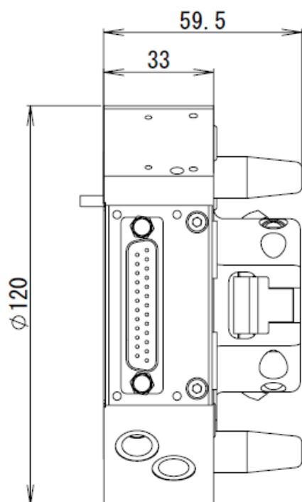
R側アダプタ (詳細は納入仕様図面参照のこと)
