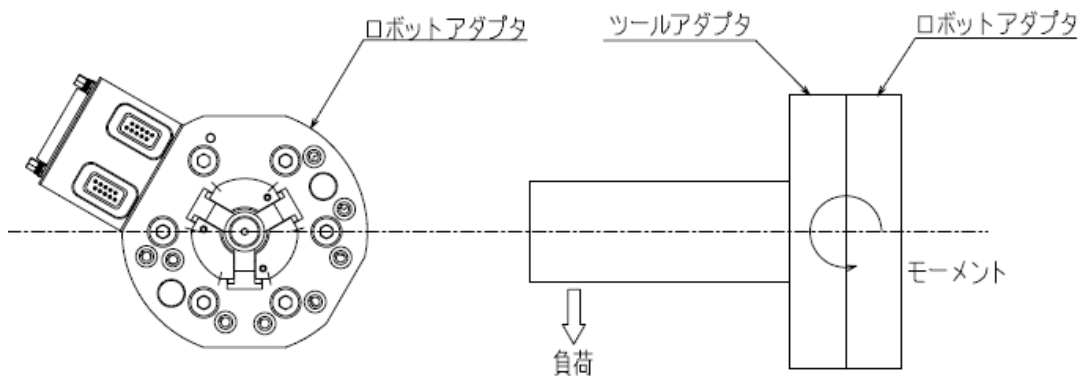
図 11. A T Cの取付方向
