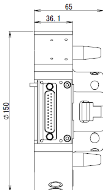
R側アダプタ (詳細は納入仕様図面参照のこと)
