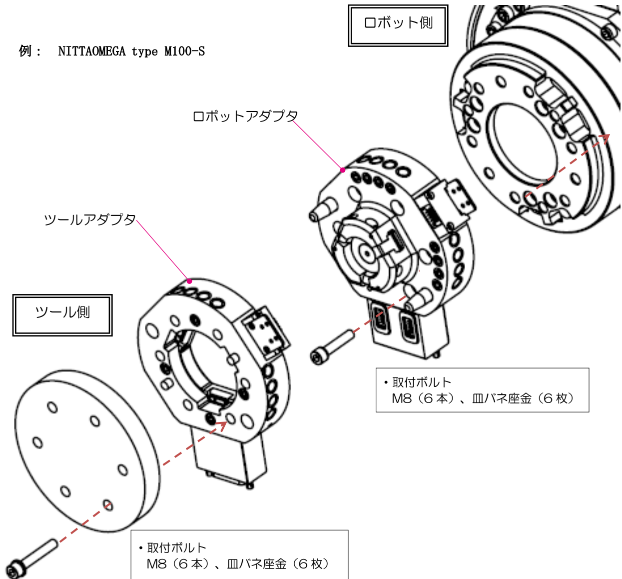
図 1. システム図
