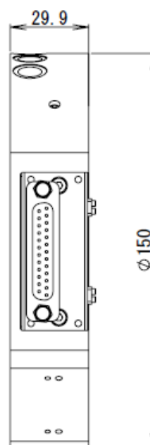
T側アダプタ (詳細は納入仕様図面参照のこと)
