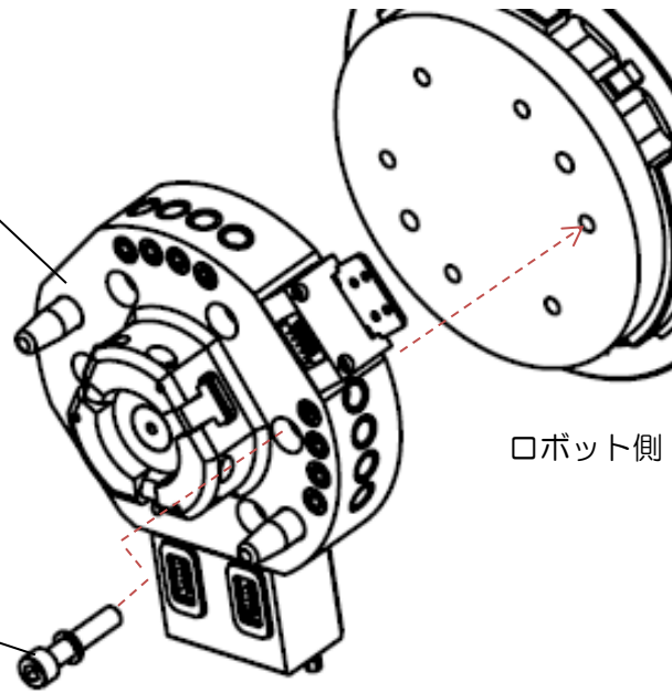
図 8. ロボットアダプタの取付
