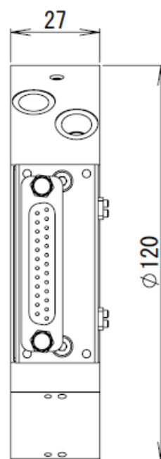
T側アダプタ (詳細は納入仕様図面参照のこと)
