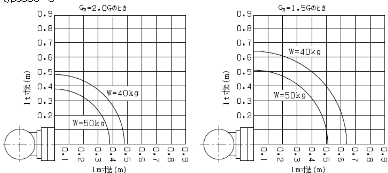
図 4. 定格負荷の定義一例 G_R=1.5, 2.0 の場合
