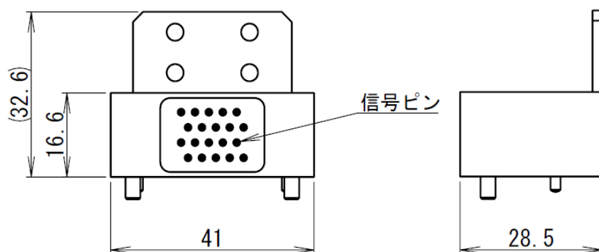
R側信号モジュール （詳細は納入仕様図面 参照のこと）
