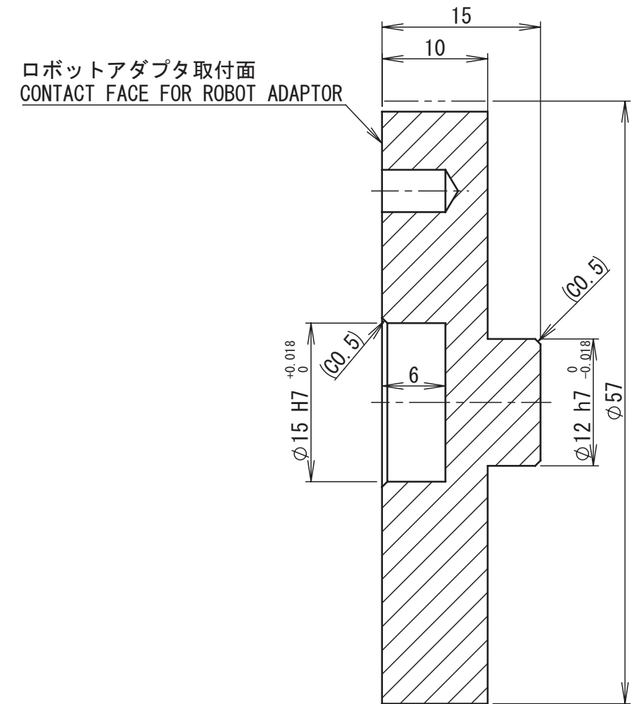
断面図 A-A SECTION A-A
