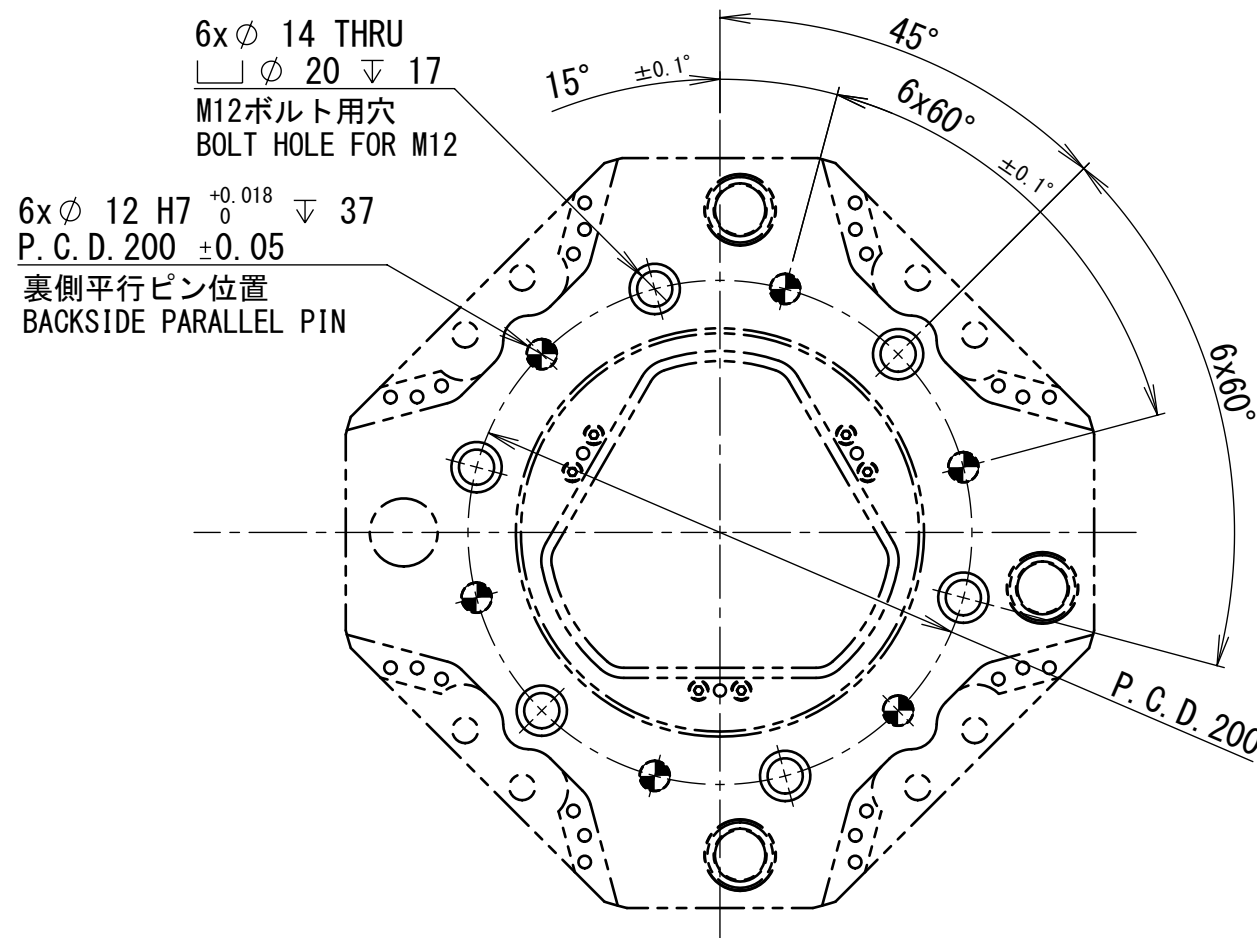
矢視図 A: 取合い寸法図 VIEW A: CONNECTING DIMENSION VIEW
