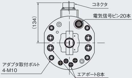
ロボットアダプタ
