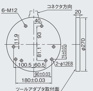
ツールアダプタプレート
