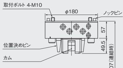
ツールアダプタ
