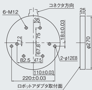
ロボットアダプタプレート
