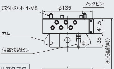
ツールアダプタ
