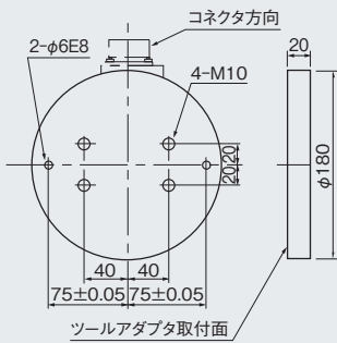
ツールアダプタプレート
