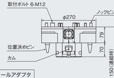
ツールアダプタ
