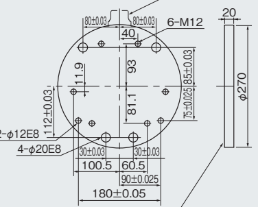
ツールアダプタプレート
