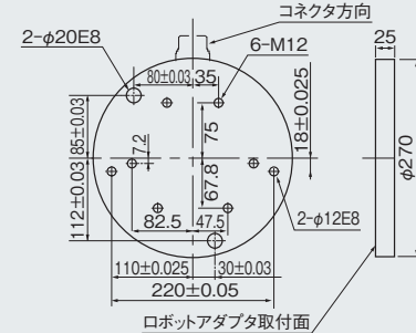
ロボットアダプタプレート
