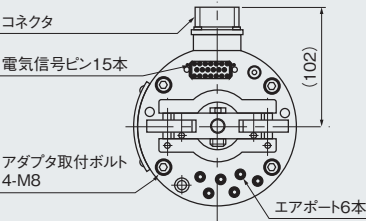
◆外形寸法図
