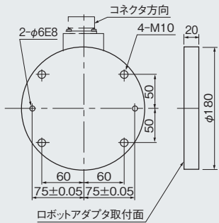
ロボットアダプタプレート
