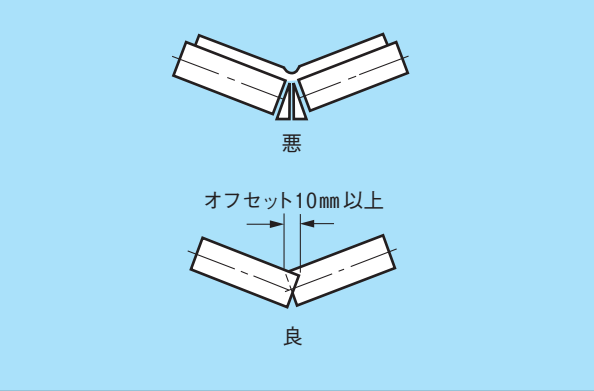
図-28 2本ローラトラフ
