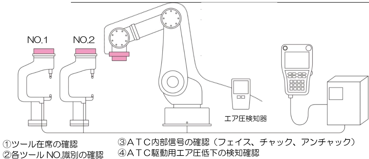
図 11. インターロックの例
