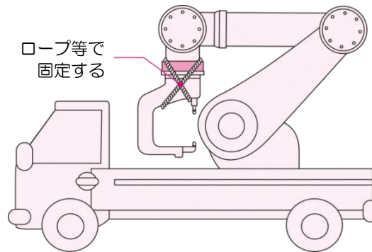
図 15. 運搬時の注意
