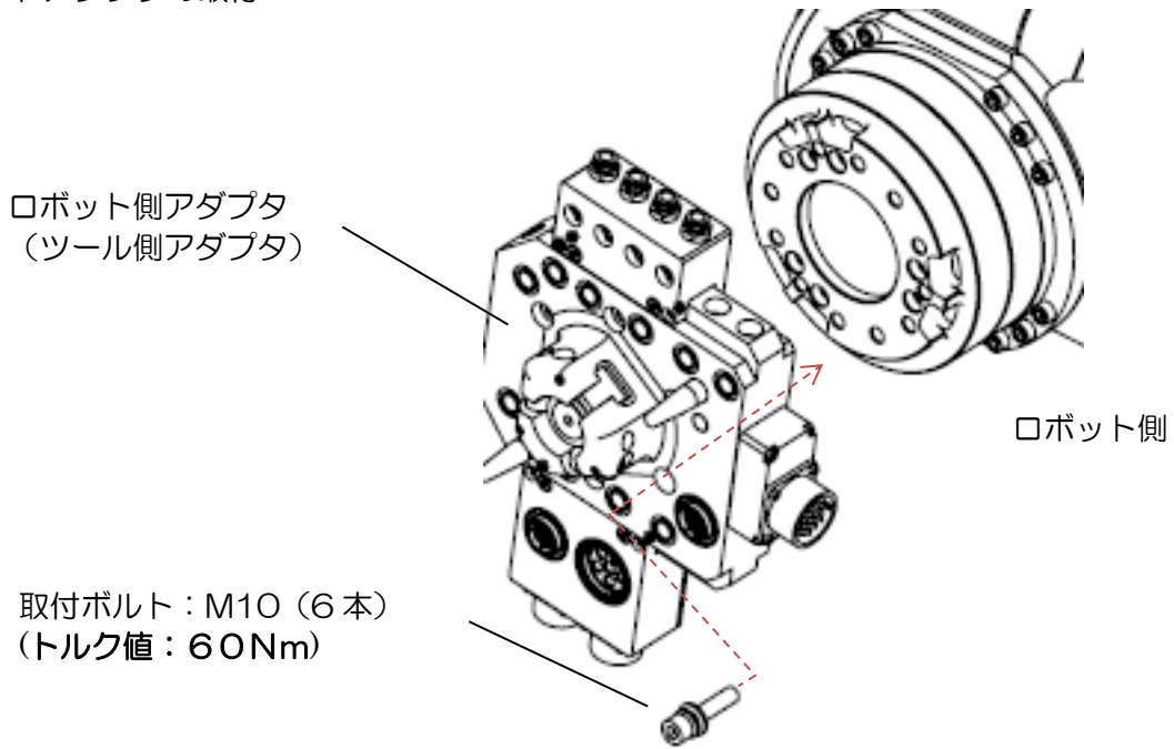
図 7. ロボットアダプタの取付
