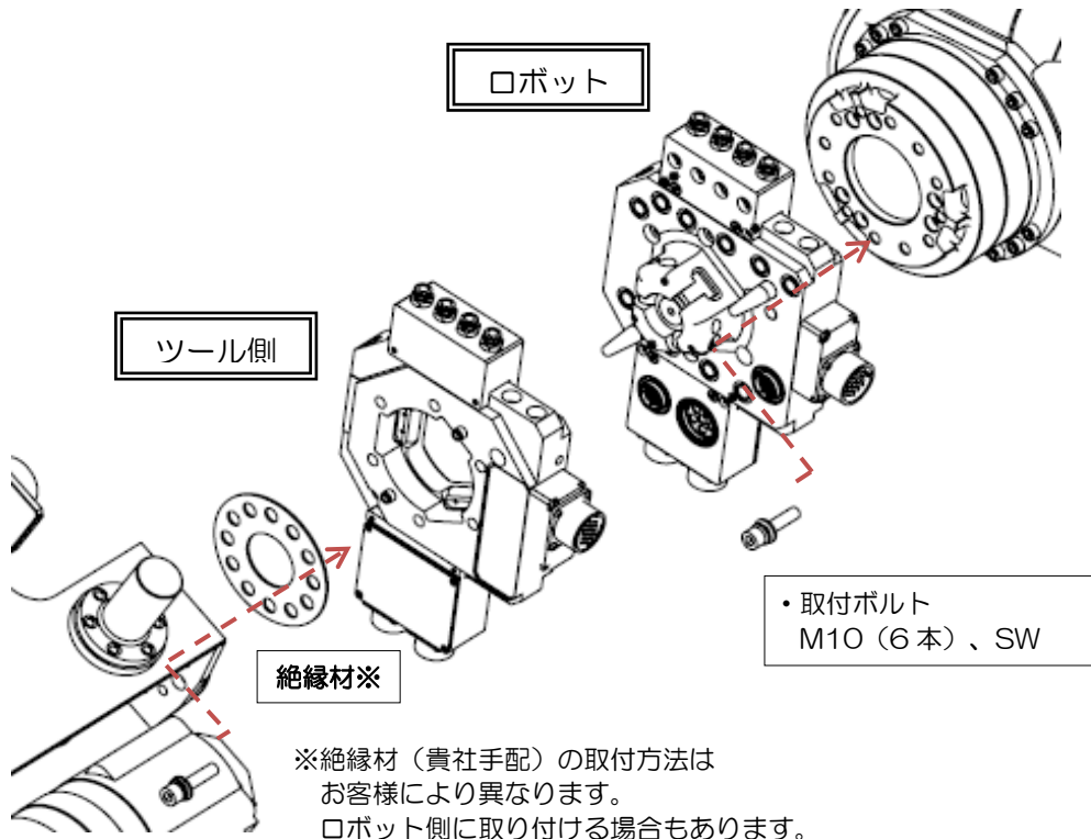
図 5. ロボットおよびツールの組立図
