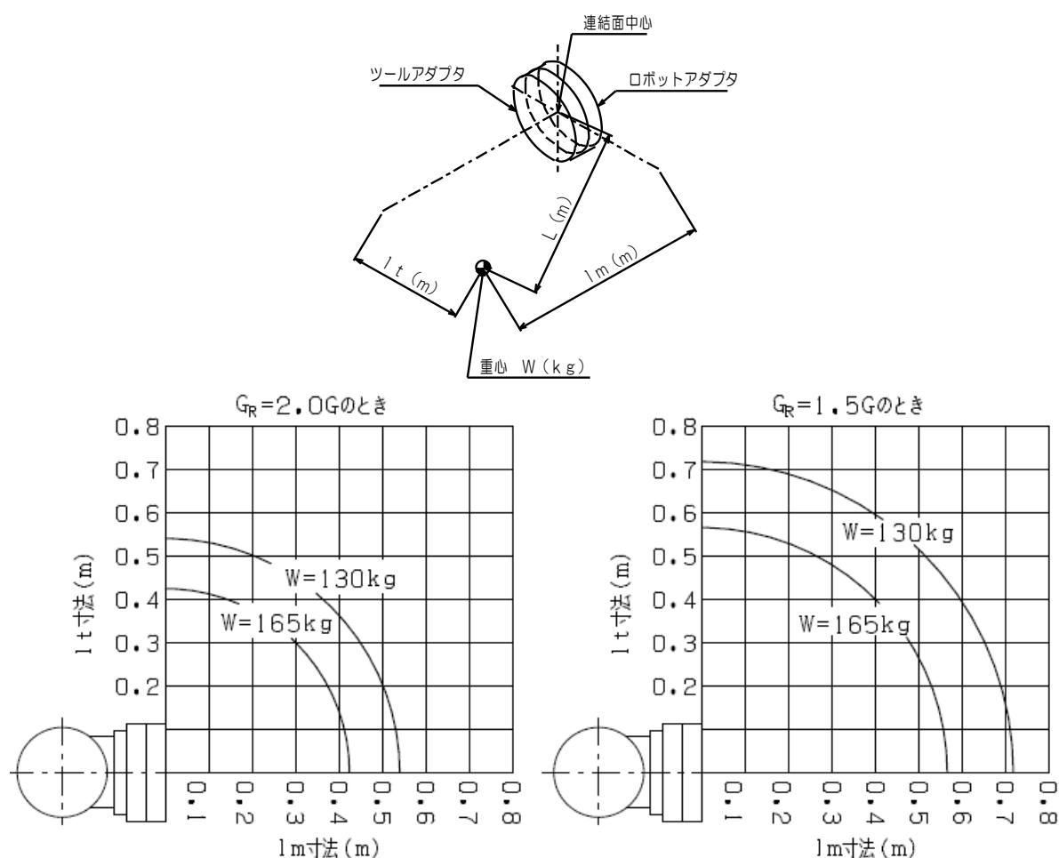
図 3. 定格負荷の定義一例 G_R=1.5, 2.0 の場合
