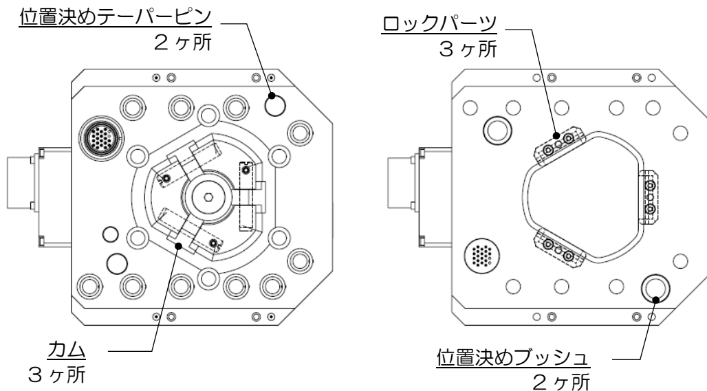
図 9. ATC給脂箇所
