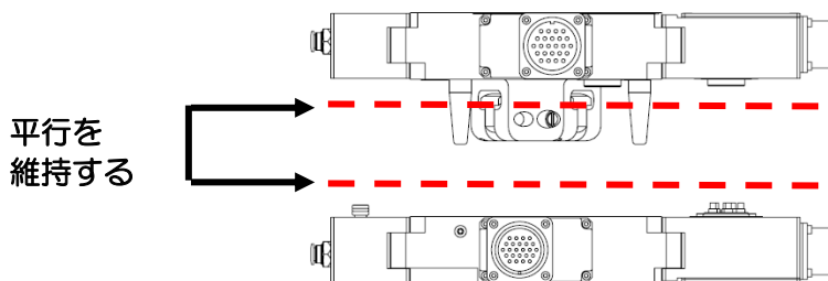
図 12. ティーチング時の注意
