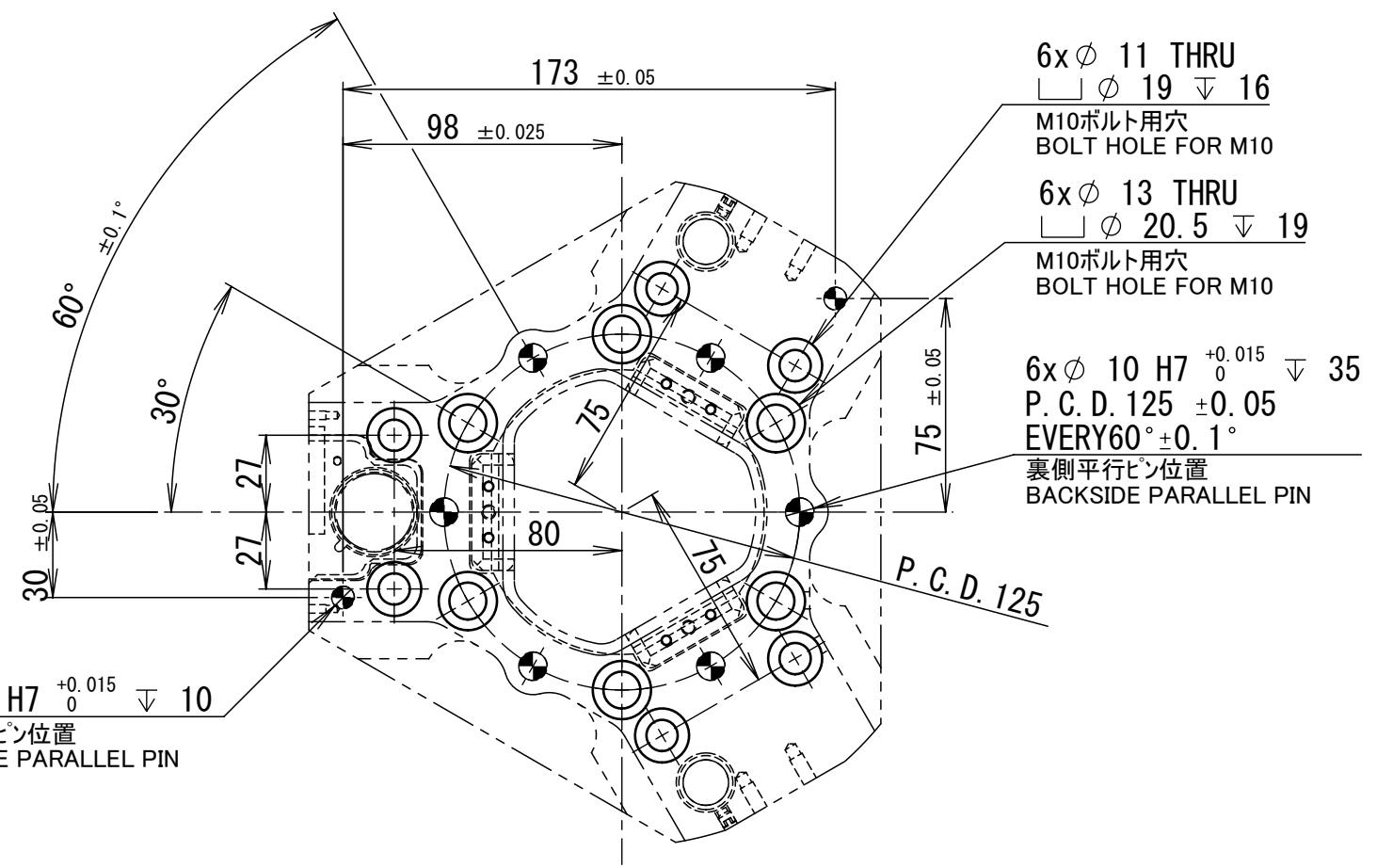
矢視図 A : 取合い寸法図 VIEW A : CONNECTING DIMENSION VIEW
